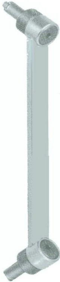
27-05-00-1600 Bohrbuchse neutral exzentrisch für Bohrer Ø 2,5mm Drill guide neutral and excentric holes for drill Ø 2,5mm
